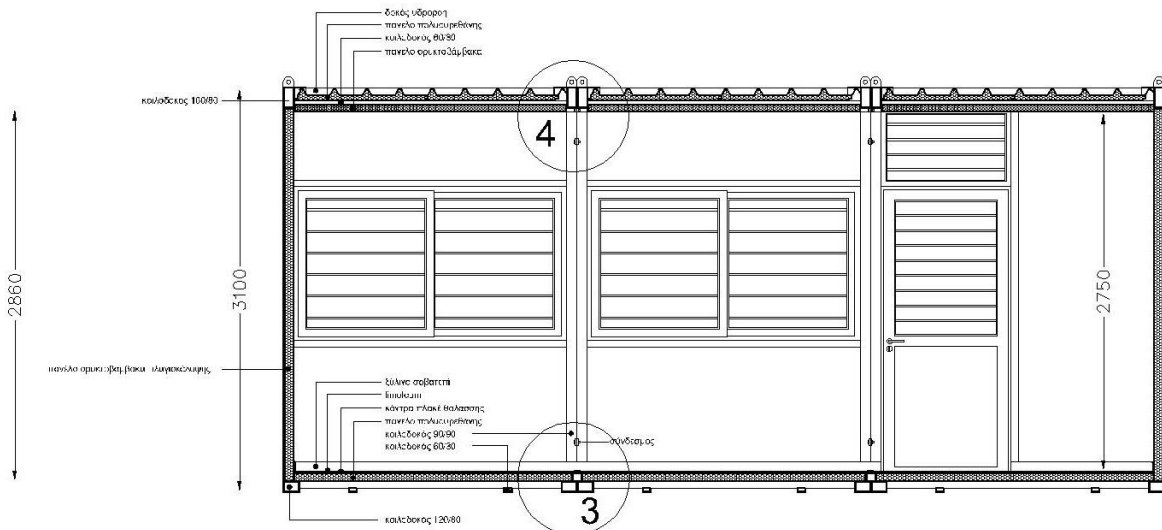
Τομή 1-1
