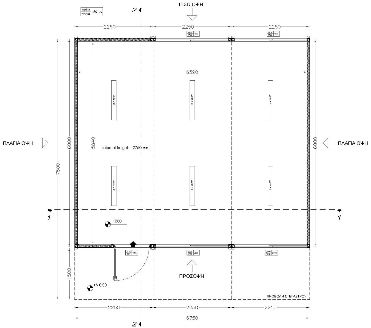
Κάτοψη Αίθουσας
